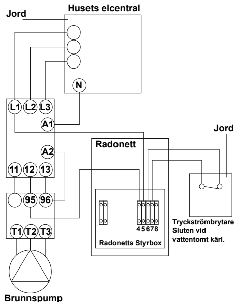
B Normal installation med Radonett utan filteranläggning
