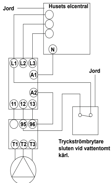
A Normal installation av brunnspump. Utan Radonett.
