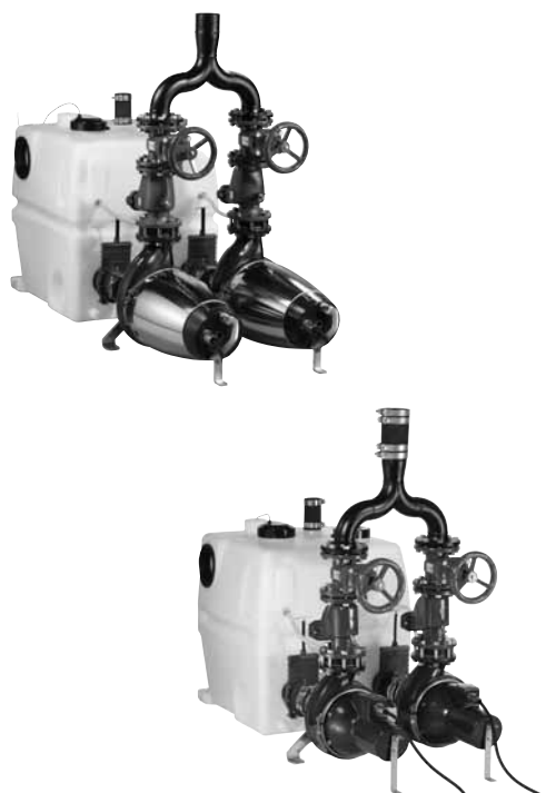
Fig. 31 Multilift MD1/MDV
