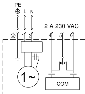
Fig. 4 Kopplingsschema, 1-faspump
