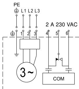
Fig. 5 Kopplingsschema, 3-faspumpar
