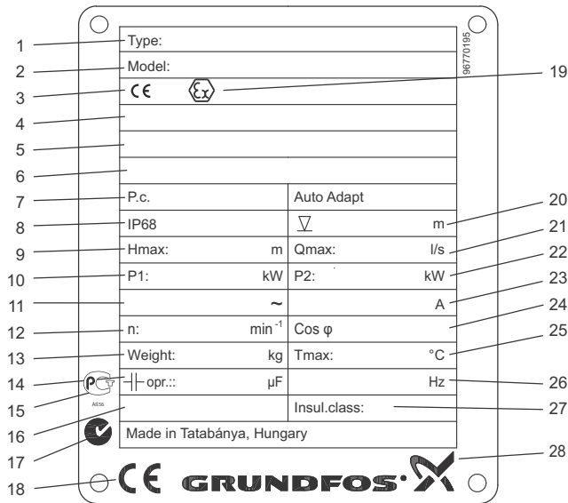
Fig. 3 Typskylt
