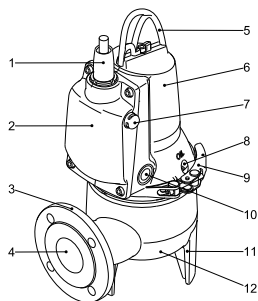
Fig. 2 Pump SLV.65.65
