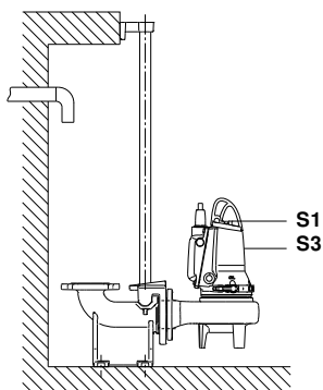
Fig. 10 Driftsnivåer
