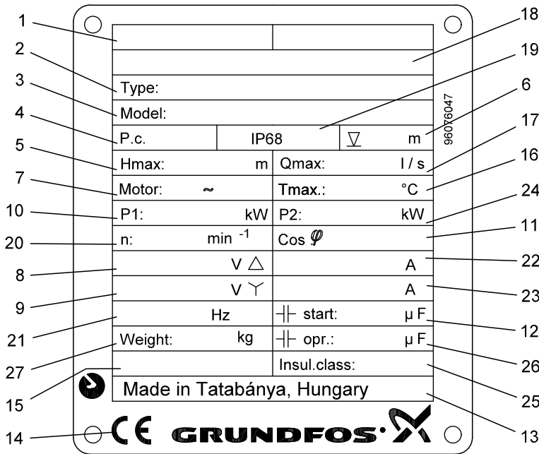
Fig. 4 Typskylt
