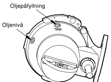
Fig. 13 Hål för påfyllning av olja
