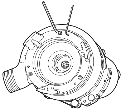
Fig. 12 Pumpen sedd från sugporten
