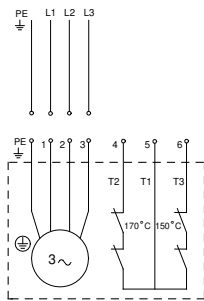
Fig. 6 Kopplingsschema, 3-faspumpar
