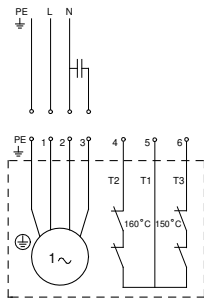
Fig. 5 Kopplingsschema, 1-faspump
