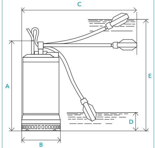
Måttkiss: SX 5-15
