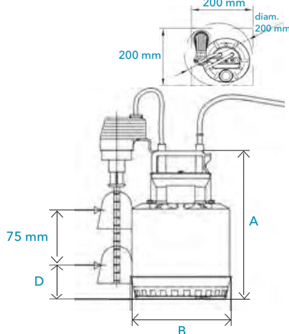
Måttkiss: SX 2-3 GW (flottör)
