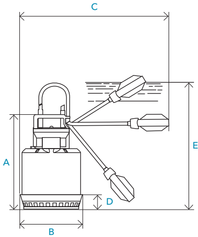
Måttkiss: SX 2-3
