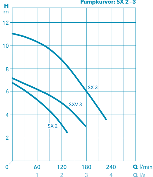
Pumpkurvor: SX 2-3
