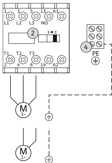
Fig. 8: Pumpanslutning
