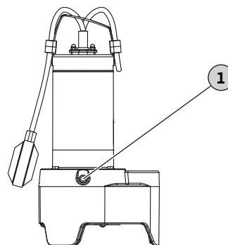
Fig. 3: Oljebyte tätningsskammare
